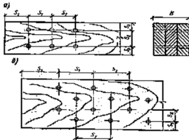
Рис. 10. Расстановка нагелей
