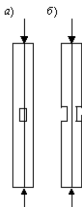
Рис. 1. Ослабление сжатых элементов
