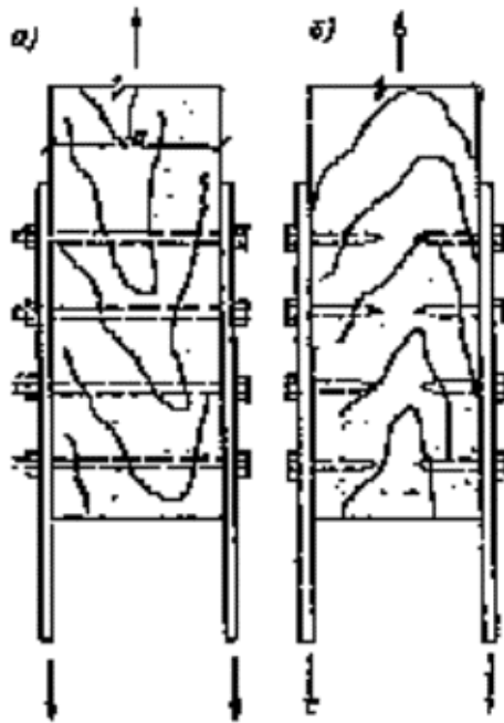
Рис. 9. Нагельные соединения со стальными накладками
