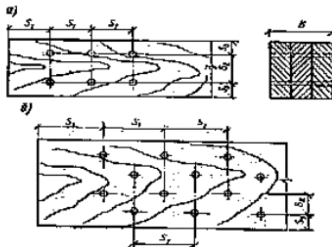
Рис. 10. Расстановка нагелей
